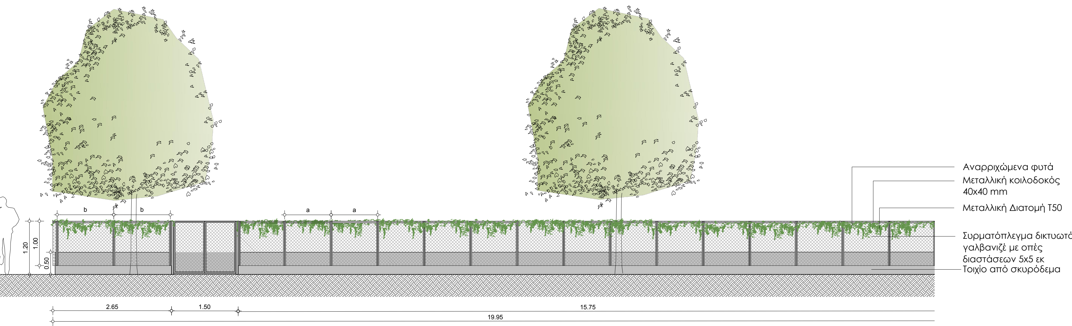
ΟΨΗ ΚΑΙΜΑΚΑ 1:50 Λ01_ΛΕΠΤΟΜΕΡΕΙΑ ΜΕΤΑΛΛΙΚΗΣ ΠΕΡΙΦΡΑΞΗΣ ΣΤΟΝ ΧΩΡΟ ΠΑΙΧΝΙΔΙΟΥ
